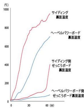
【外壁材裏面と内装せつこうボード裏面の温度変化】
